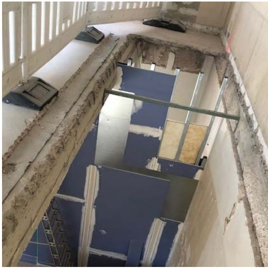
Juni: Durchbruch der Decken
